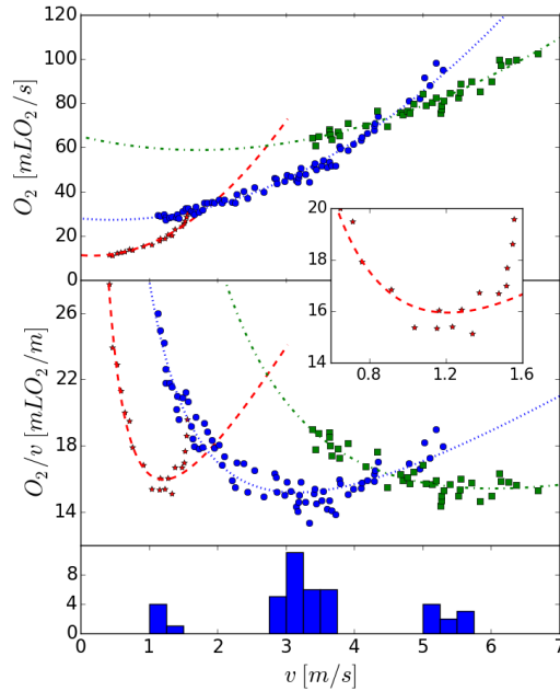
FIGURE 1 – Flux de consommation en oxygène O_2 (en haut), COT = O_2/v (au milieu), dans le cas du déplacement d'un cheval aux trois allures : pas, trot et galop. On notera (histogramme du bas) que les vitesses préférentiellement choisies par l'individu laissé libre coïncident avec les minimas du COT pour chaque allure. Les courbes sont les ajustements aux données expérimentales, réalisés par le modèle thermodynamique, extrait de [3].
